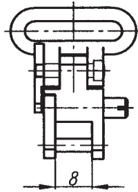
SECURA-Riemenbügelkörper mit EURO-Öse Bestell-Nr. 22011-1000
