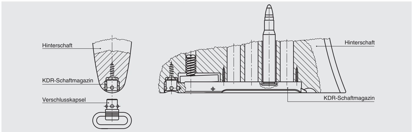
Schaftmagazin aus Stahl für vier Patronen mit KDR-Verschluss zum Einpassen in den Hinterschaft. Guter optischer Gesamteindruck.
