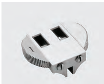
Schlösschen für Drillinge, mit konisch vorgefrästen Radien.
