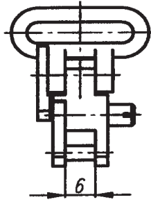
SECURA-Riemenbügelkörper mit EURO-Öse Bestell-Nr. 22009-1000
