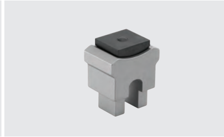
Hinterfüsse, für S&B-Convex-Schiene, ohne Support; kurze Ausführung.
