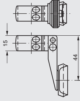
ERAMATIC- Schwenkmontagen mit Klemmringsen aus Stahl ø 34 mm Verlängerung: 44 mm Bauhöhe: 18,5 mm
