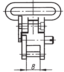
SECURA-Riemenbügelkörper mit US-Öse Bestell-Nr. 22011-3000
