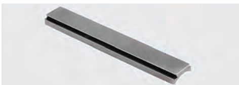
Schienenstück mit 30°-Prisma für BBF. Prisma passt für R6, H7, G9 und G9-PLUS-Verschlusskörper. Länge: 110,0 mm, Bauhöhe: 3,5 mm
