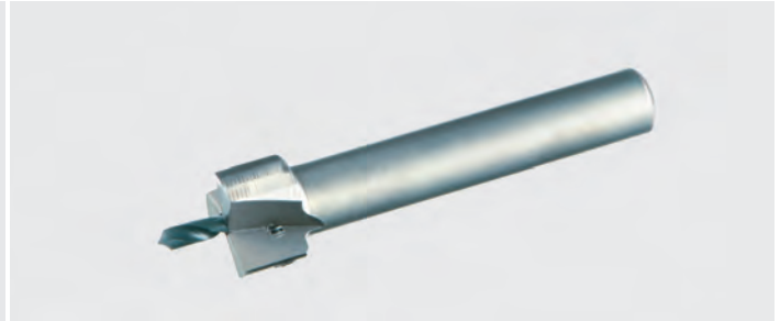
Mit dem Zapfensenker lässt sich die Bohrung für den äusseren Durchmesser der KDR-Buchse im Schaft herstellen. Der Spiralbohrer stellt den Kerndurchmesser für die Holzschraube her. Die Tiefe muss nachgebohrt werden.
