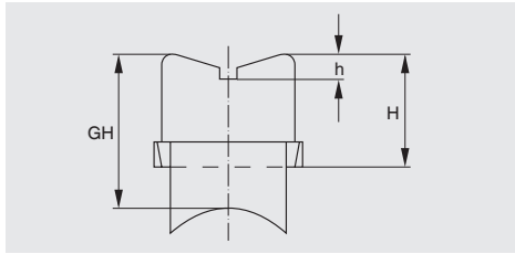
Gesamthöhe: GH = H + 5 \text{ mm}
