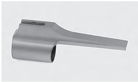
Ringkornsattel mit Längsprisma, ohne seitliche Rillen, aus einem Stück gefertigt, flache Sichtfläche. Breite: 9 mm; BH: 9 mm
