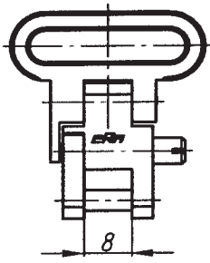
SECURA-Magnum Riemenbügelkörper
