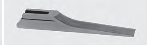
Kornsattel mit Längsprisma und gerundeter Sichtfläche. Radius: 7,5 mm; Breite: 10 mm; BH: 8 mm 12010-0000
