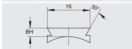
Basen für Aufkippmontagen mit 16 mm Prisma; Vorderbasen BH 3,5 mm; Höhe der Hinterbasen ist modellbezogen.
