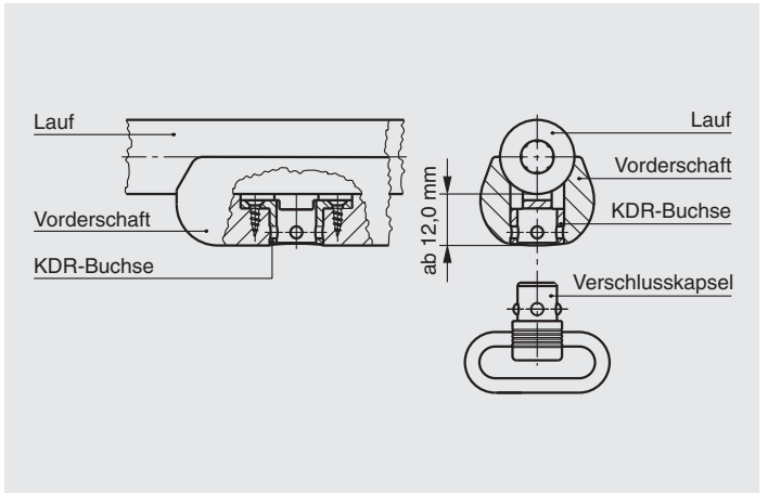
Kugeldruckriemenbügel-Buchse für besonders schlanke Vorderschäfte, mit zwei Holzschrauben von innen angeschraubt.
