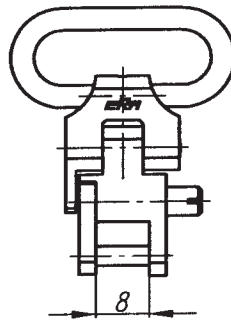
SECURA-Riemenbügelkörper mit eingebogener Drahtöse
