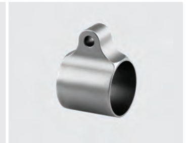
Ringriemenbügel in besonders schlanker Ausführung, zylindrisch. Kopfbreite: 8 mm; Bohrung: ø 3,6 mm.
