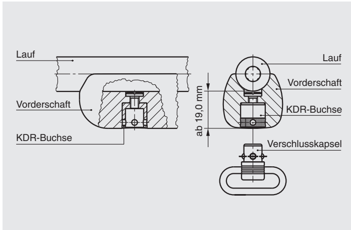
Kugeldruckriemenbügel-Buchse für schlanke Vorderschäfte, von innen angeschraubt.
