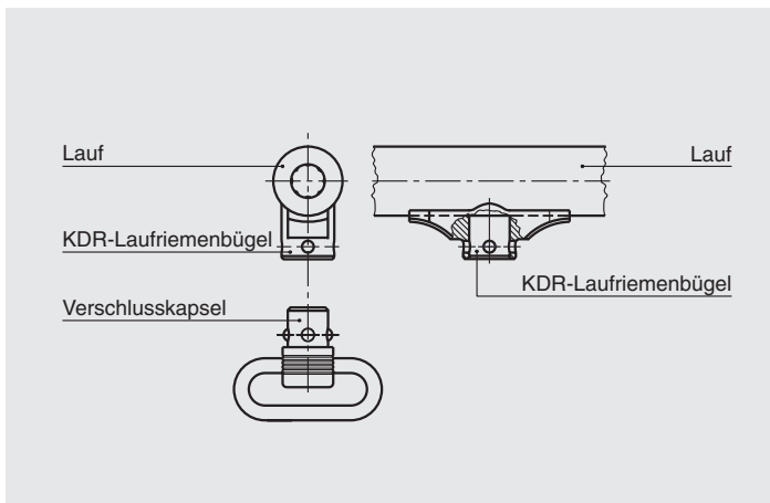
Kugeldruck-Laufriemenbügel konkav zum Anlöten an Büchsenläufe. Radius 7,5 mm
