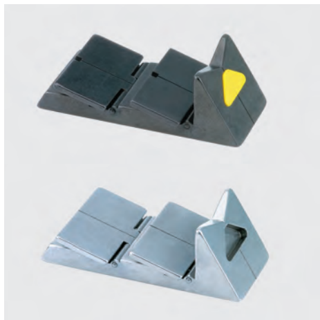
Superplus-Express-Visiere in brüniert und weißfertiger Ausführung. Prisma 30° / Länge 35,5 mm / Breite 18 mm
