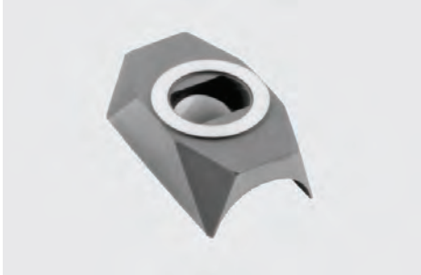
Laufsockel mit zylindrischen Radien und Drehkranz für Pivotzapfen. Radius unten geschlossen. Bauhöhe: 6,5 mm, Länge: 38 mm
