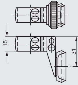
ERAMATIC- Schwenkmontagen mit Klemmringsen aus Stahl ø 34 mm Verlängerung: 31 mm Bauhöhe: 18,5 mm
