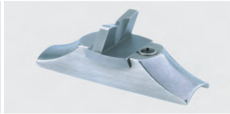
Visiereinheit bestehend aus Visiersattel mit Klemmscheibe, Schraube und Visier mit 16 mm Prisma. Der Visiersattel kann angeschraubt und/oder gelötet werden.
