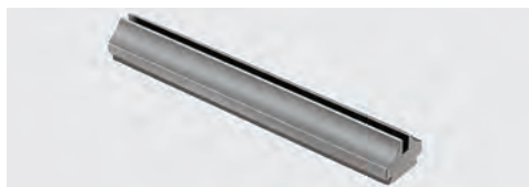
Schienenstück mit 30°-Prisma für Drillinge. Prisma passt für R6, H7, G9 und G9-PLUS-Verschlusskörper. Länge: 110,0 mm
