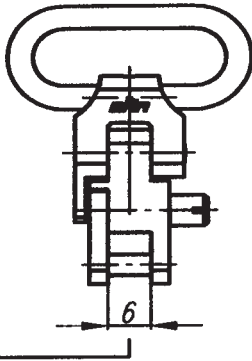
SECURA-Riemenbügelkörper mit eingebogener Drahtöse
