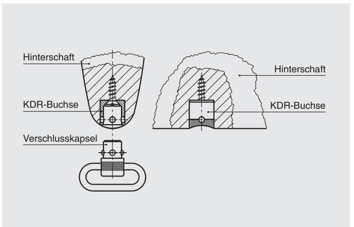
Kugeldruckriemenbügel-Buchse für den Hinterschaft mit hochgezogener, gerundeter Aussenwandung. Keine überstehenden Kanten. Passt sich harmonisch an.
