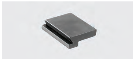
Schieneplatte mit 20°-Prisma, Anschlag und angeschrägten Stirnseiten, zum Einpassen in Laufschienen. Für V8-Verschlusskörper. Länge: 22 mm, Bauhöhe: 2,7 mm
