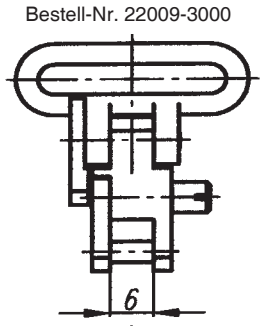
SECURA-Riemenbügelkörper mit US-Öse Bestell-Nr. 22009-3000
