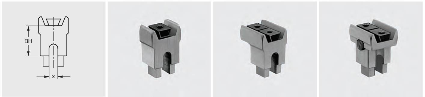
Hinterfüsse, mit 45°-Aufnahmeprisma, ohne Support; kurze Ausführung.
